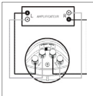
Rys. 5a Okablowanie dla wszystkich modeli (z wyjątkiem P80-SM).
